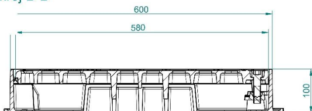
Przekrój B-B
