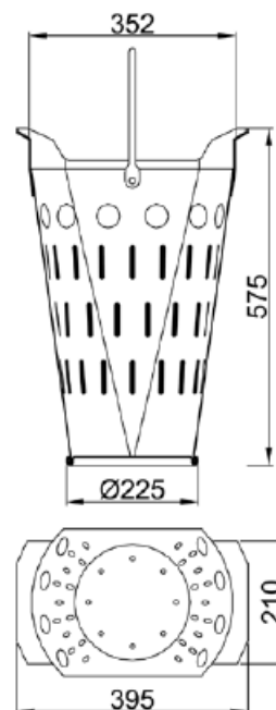
Rysunek 4 Kosz owalny typ C-3 wysoki
